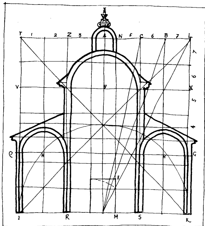
Corte transversal de uma capela, com o respectivo traçado regulador, desenhado por Philibert Delorme.
