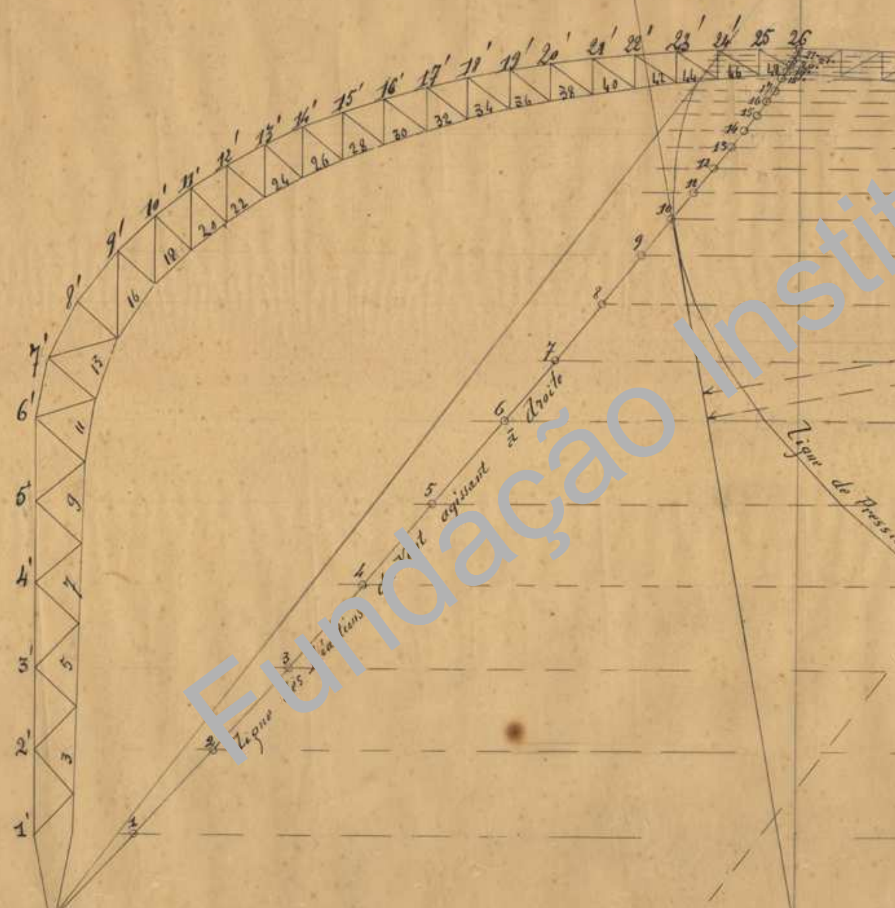
Fig 9 Polygone des Forces pour les Efforts du Vent.
