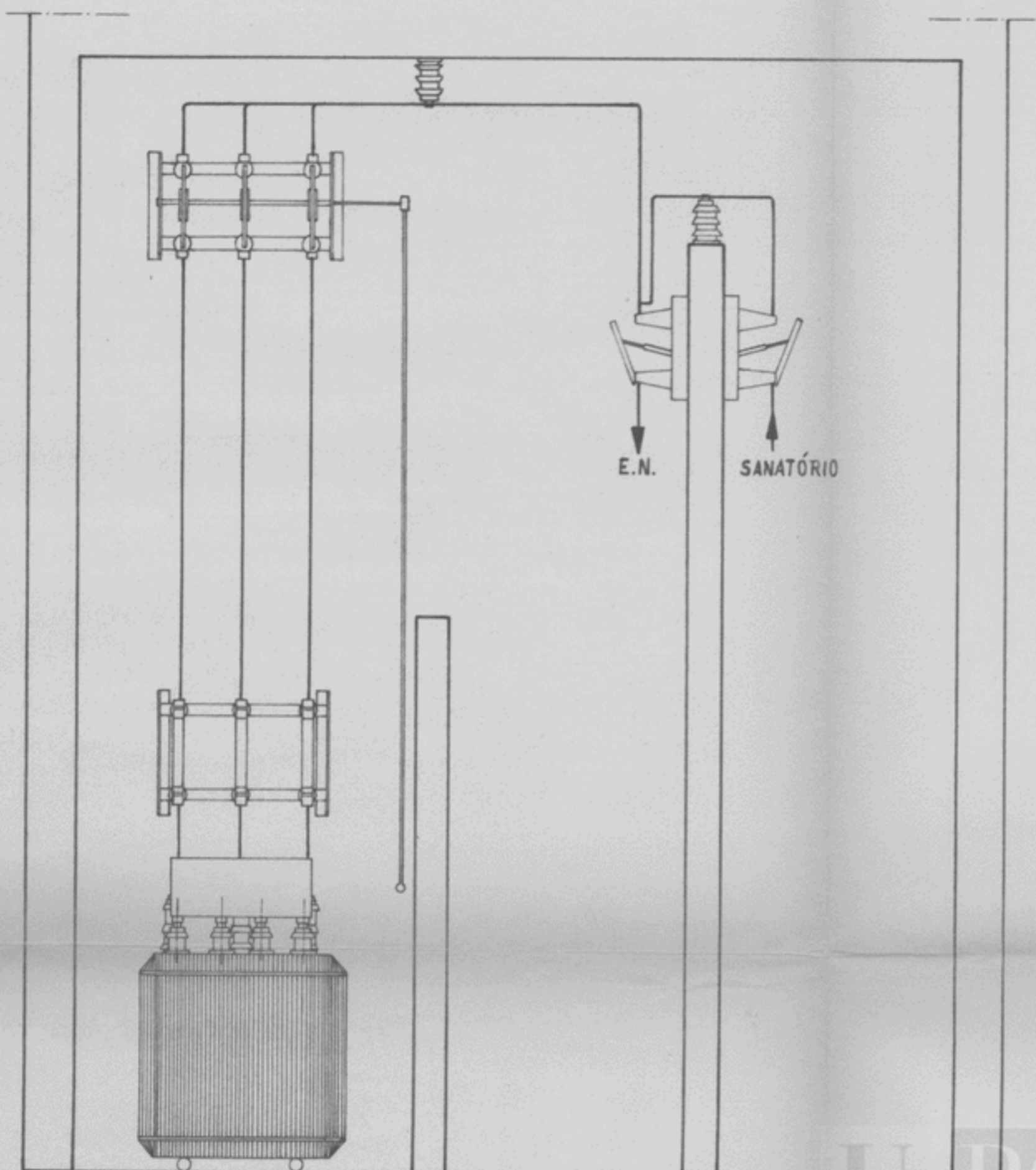
CORTE A-A'
