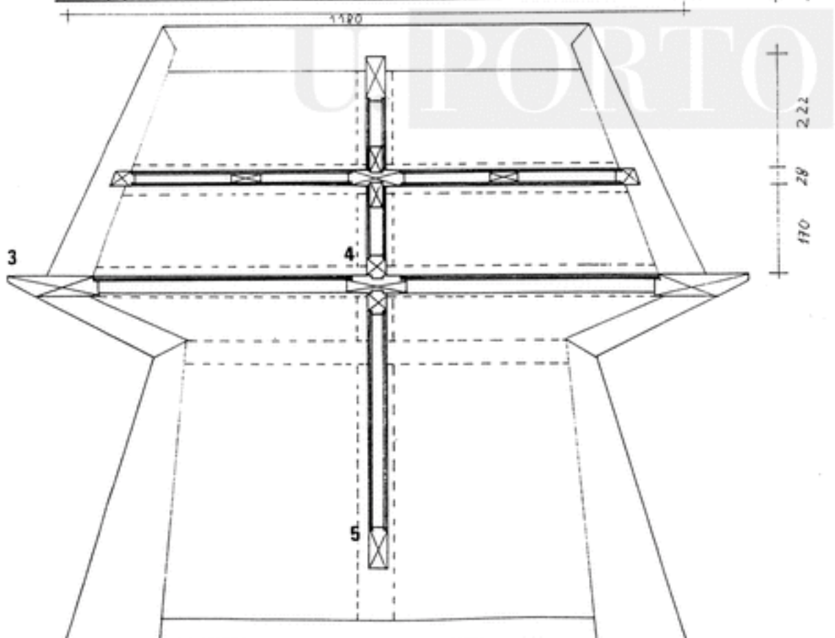
CORTE G 1
