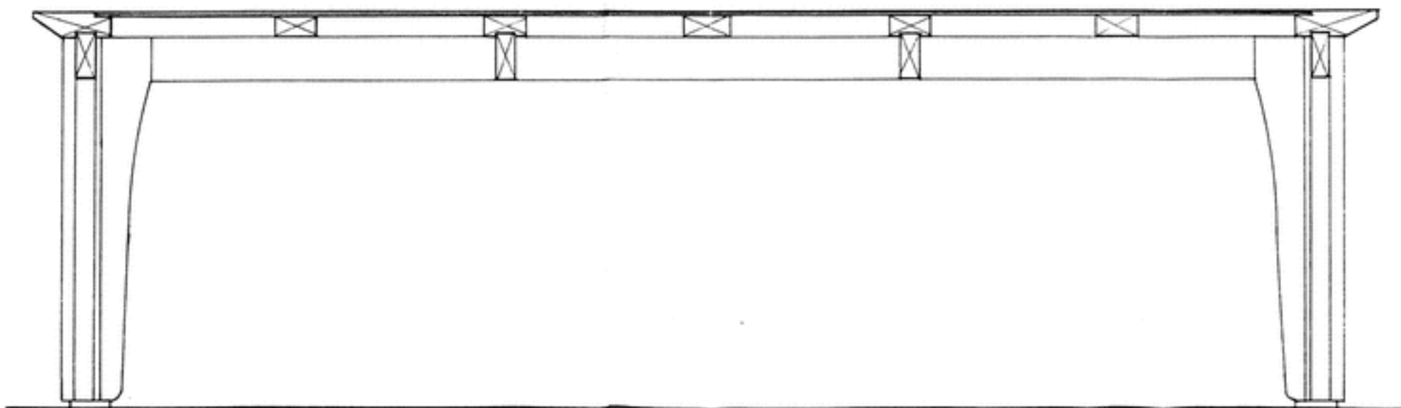
M10 : CORTE LONGITUDINAL
